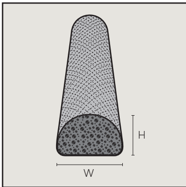
Leitfähige Dichtung – Drahtgeflecht über Elastomer.
