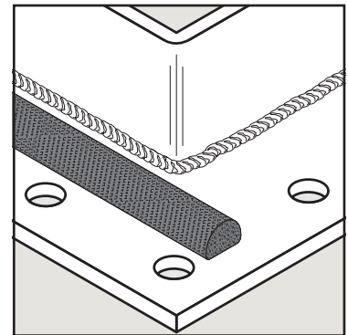
Befestigen Sie die selbstklebende Dichtung am Flansch.
