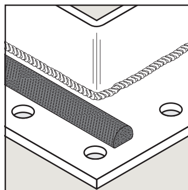
フランジ上にガスケットを取り付けます。
