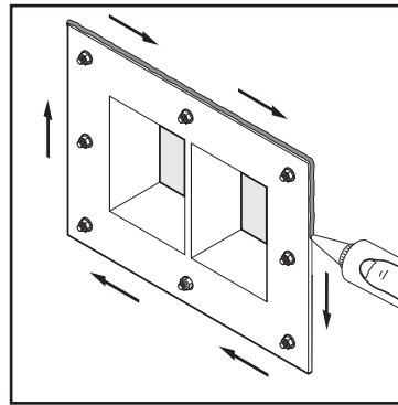
Image 5. Mastic appliqué.
